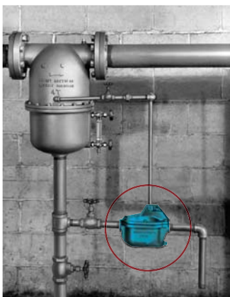
Type 230-AC Installation
